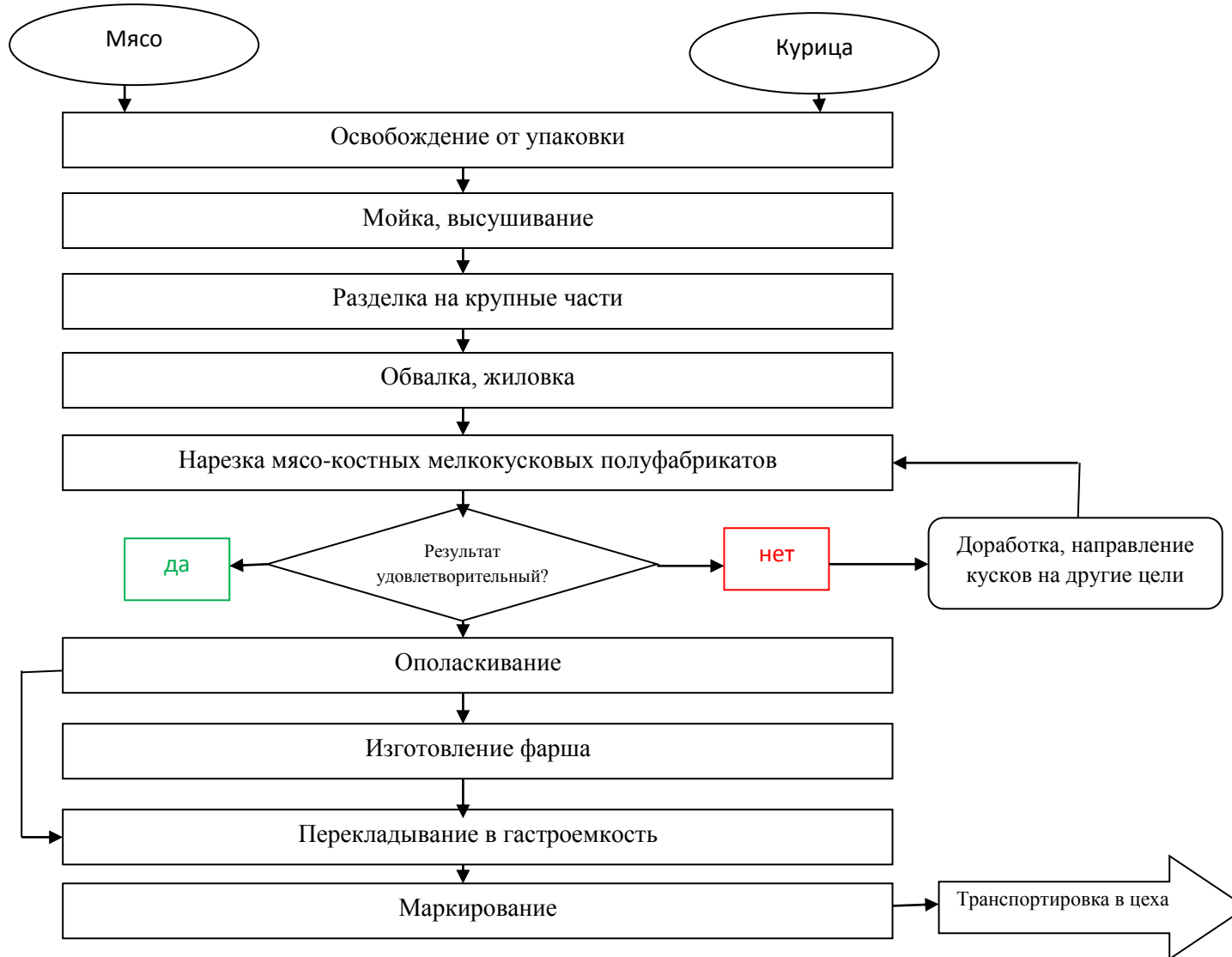
Блок-схема ТП 3.3. Технологический процесс разделки мяса, курицы
