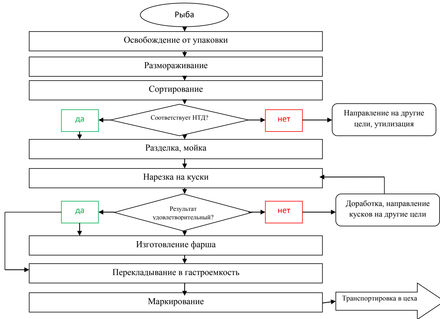
Блок-схема ТП 3.4. Технологический процесс разделки рыбы
